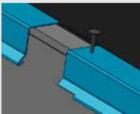
Venstre hjørneafklip på profiler
