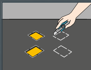
Opmærk og skær isolering.
