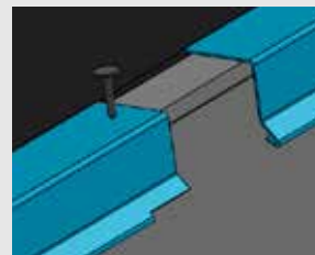
Højre hjørneafklip på profiler
